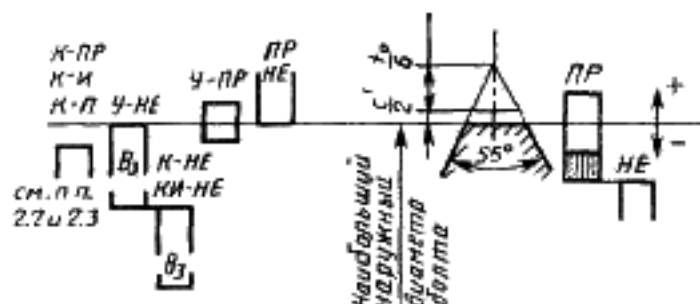
Калибры для контроля болтов (наружной резьбы)
