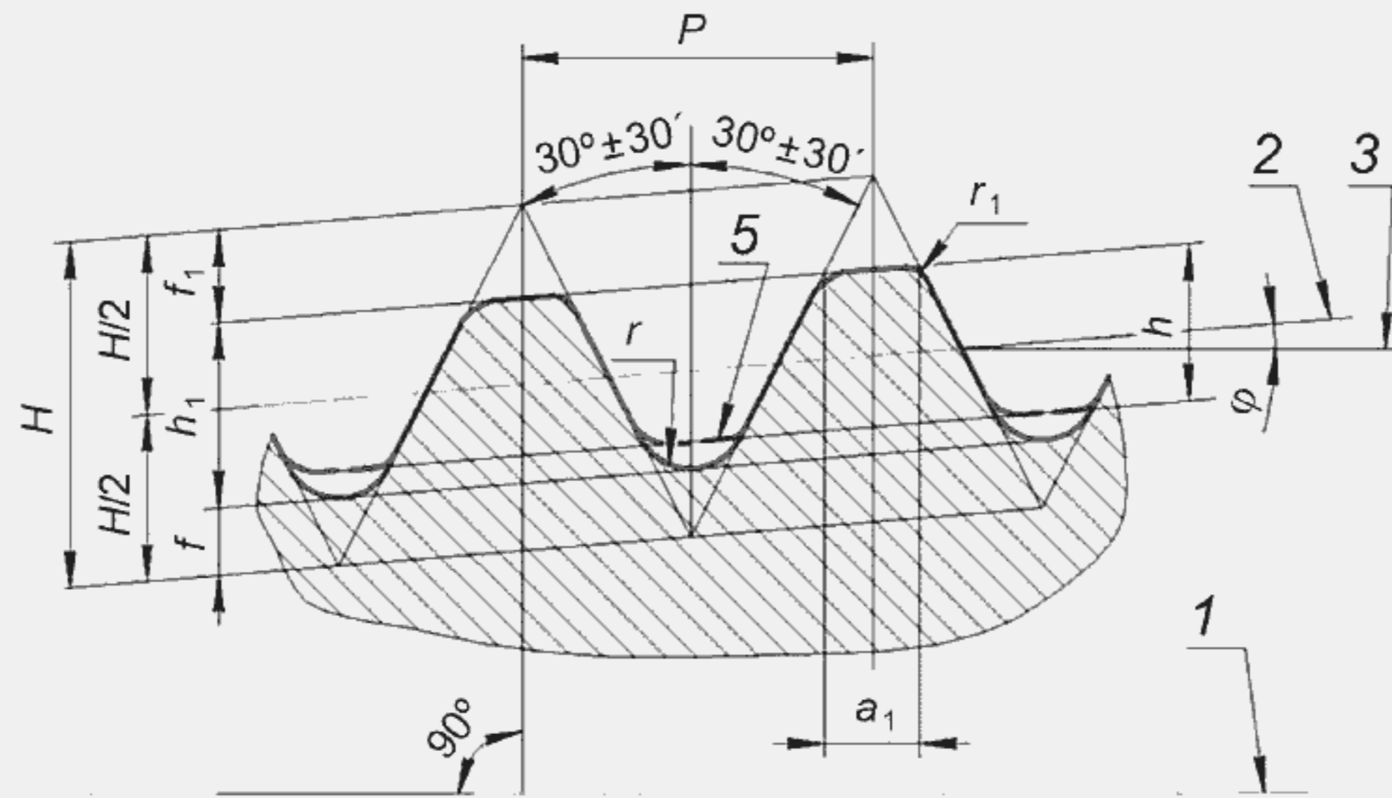
б – Профиль резьбы ниппельного конца
