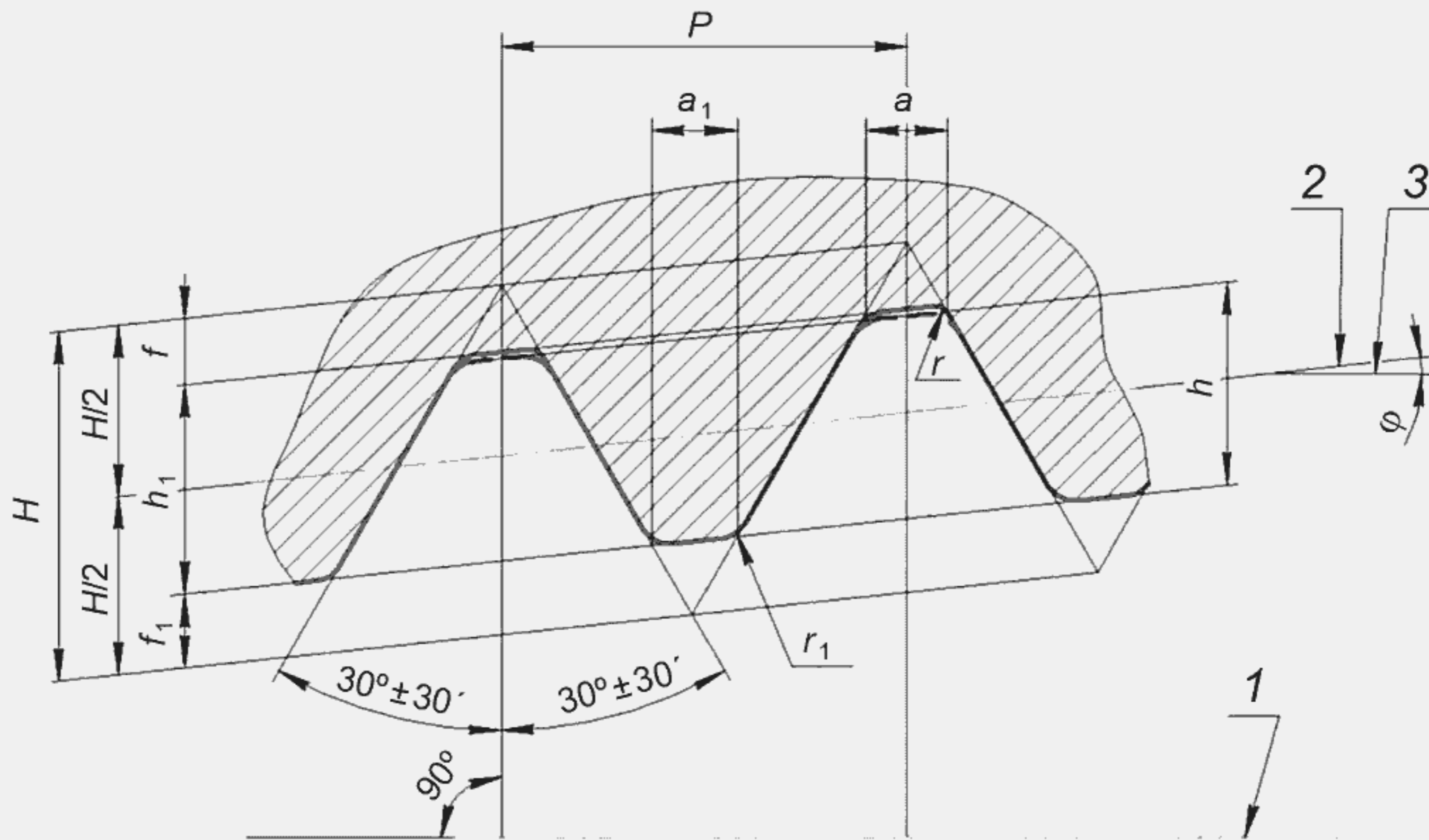
а – Профиль резьбы муфтового конца
