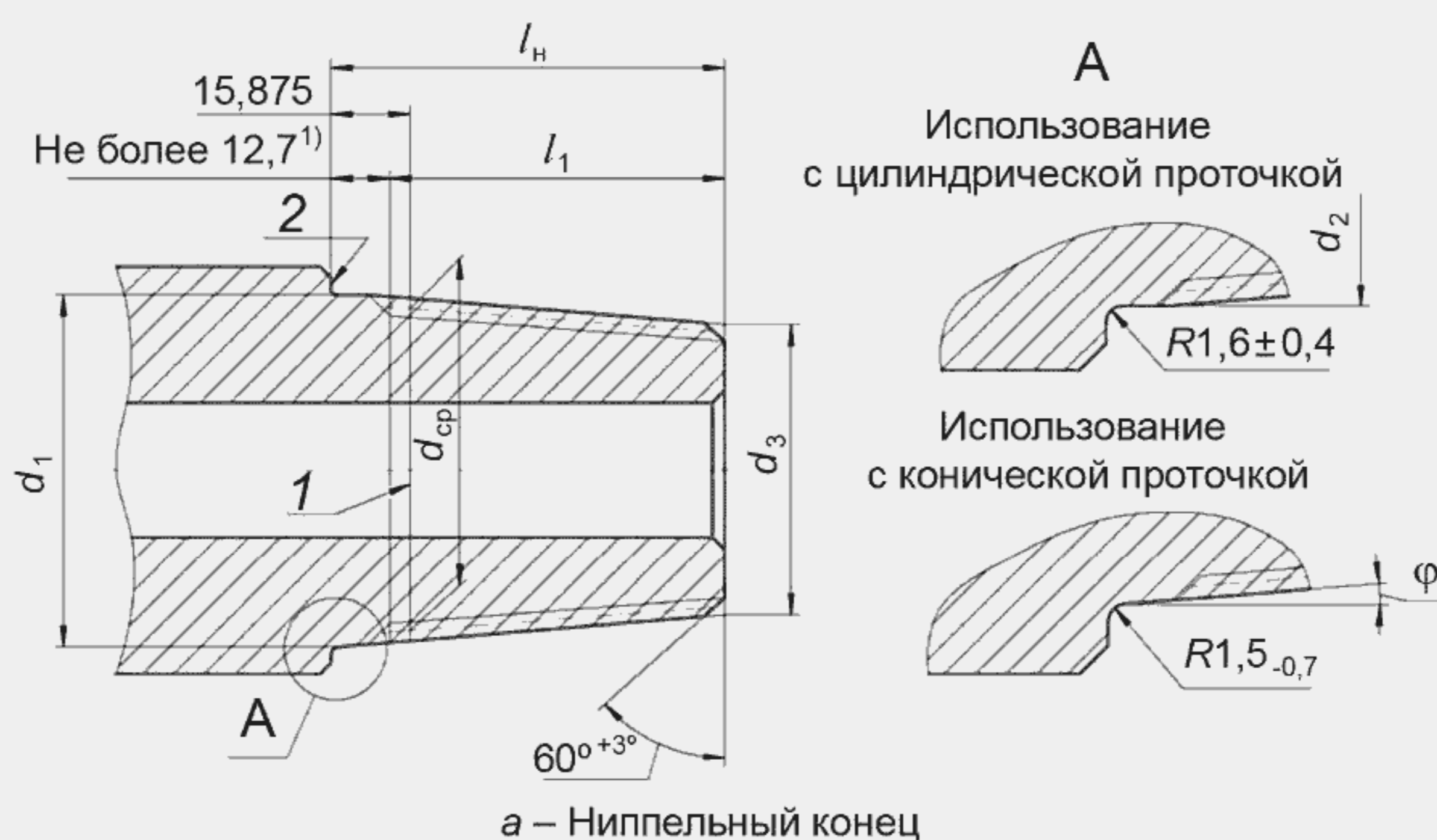
Рисунок 3 — Резьбовые соединения ниппельного и муфтового концов (Лист 1)
