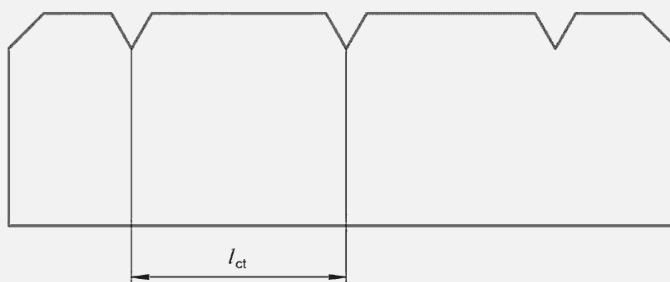
l_{ct} — компенсированная длина резьбы
