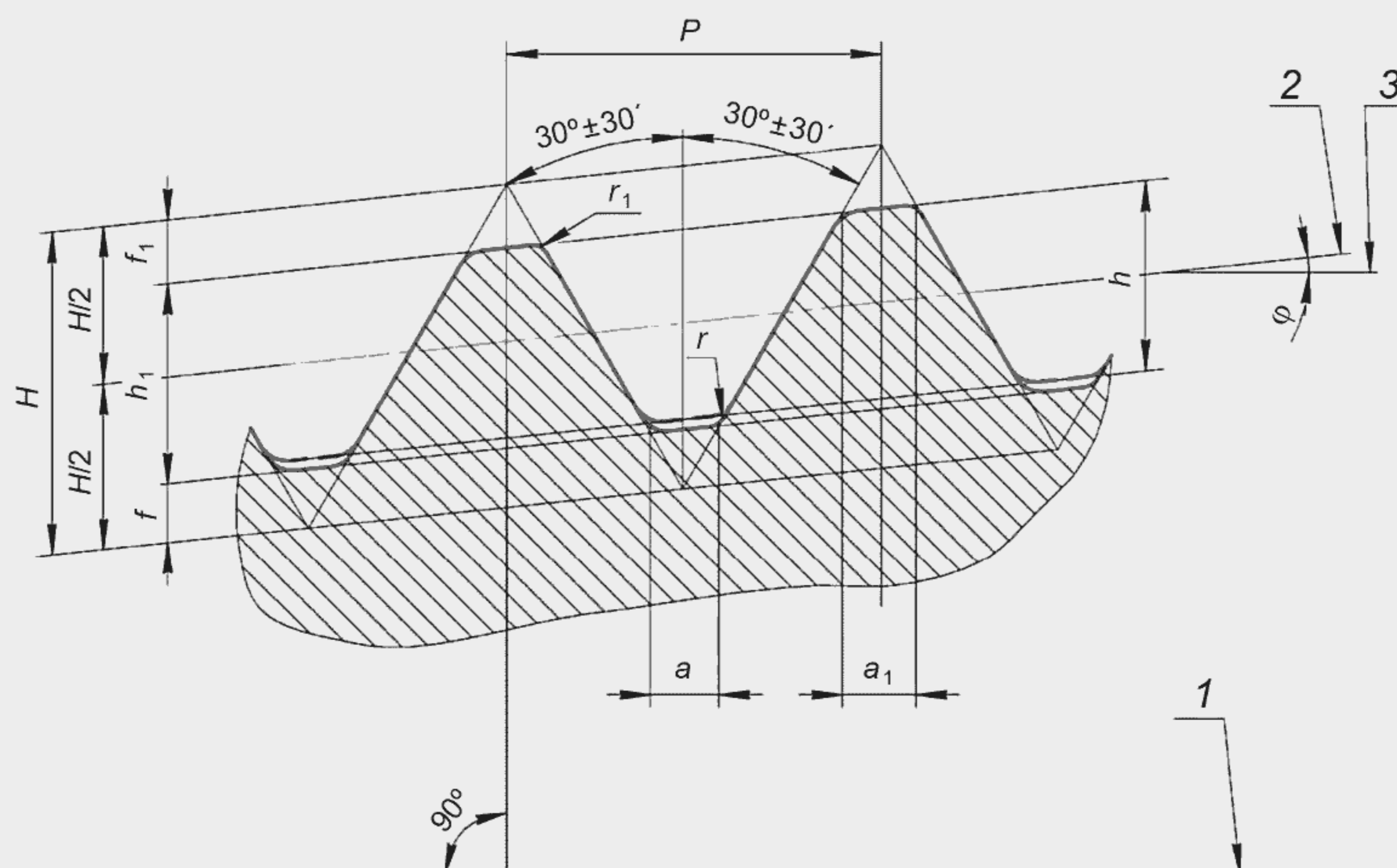
б – Профиль резьбы ниппельного конца
