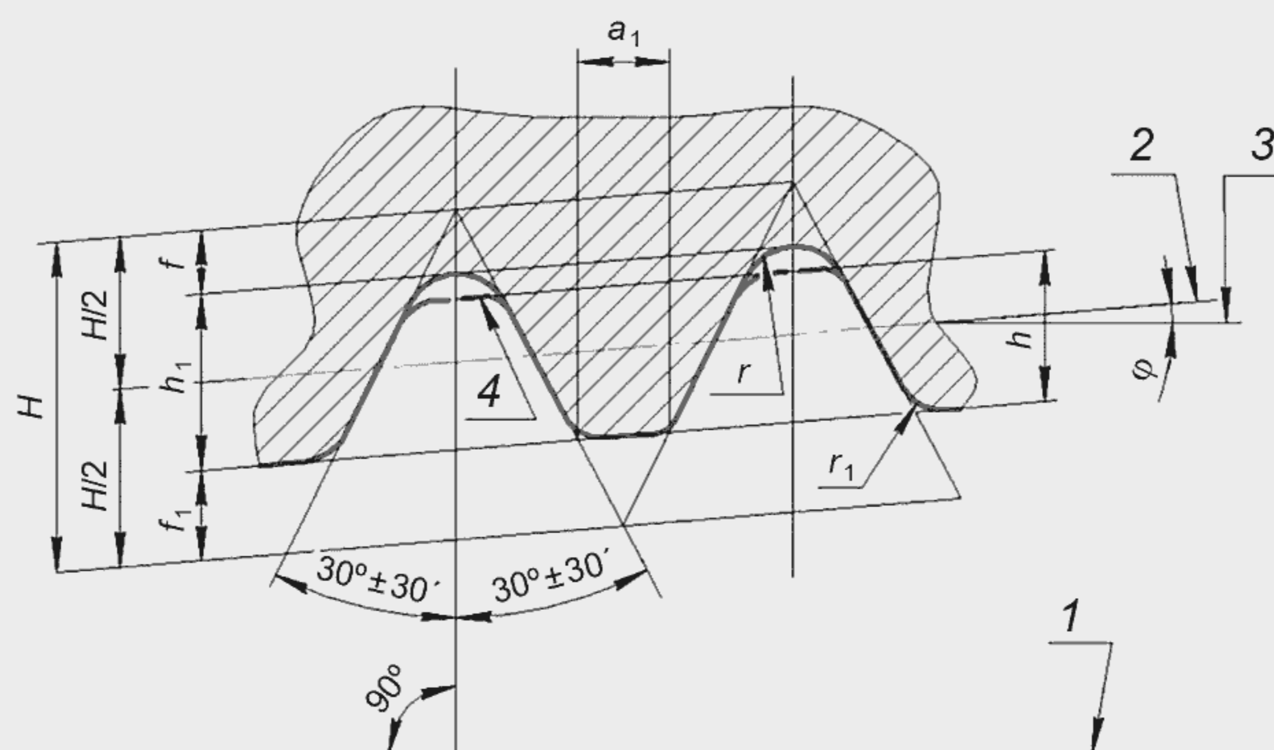
а — Профиль резьбы муфтового конца
