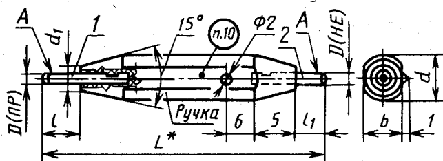
Калибр-пробка двусторонний
