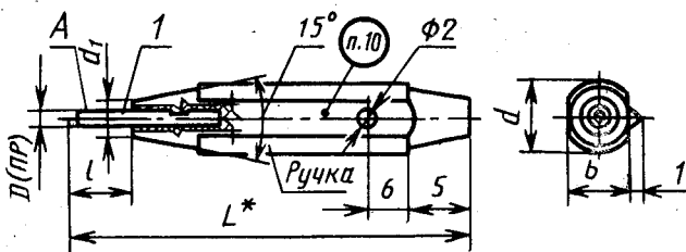
Калибр-пробка односторонний
