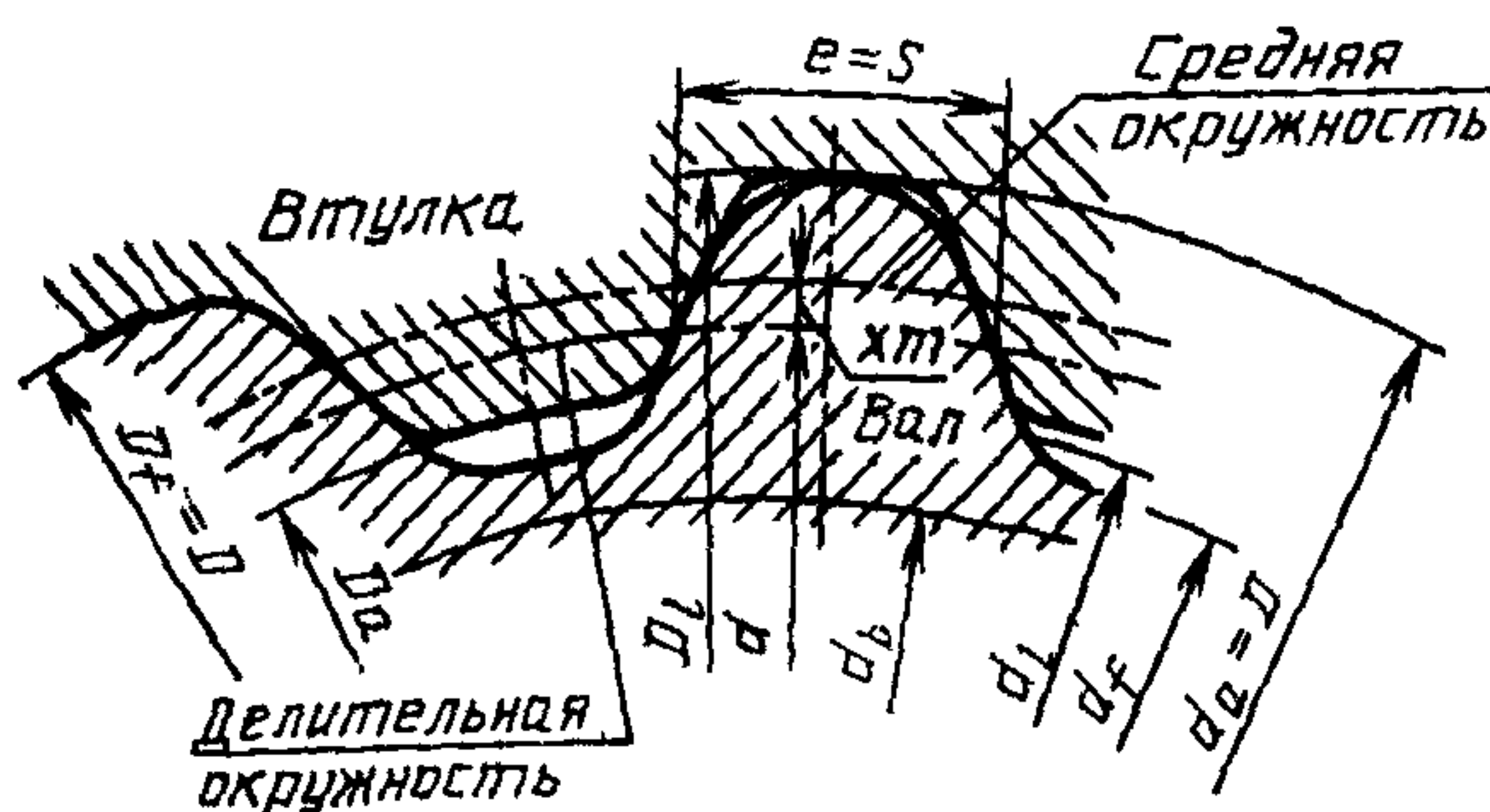
б) Форма зубьев вала и втулки
