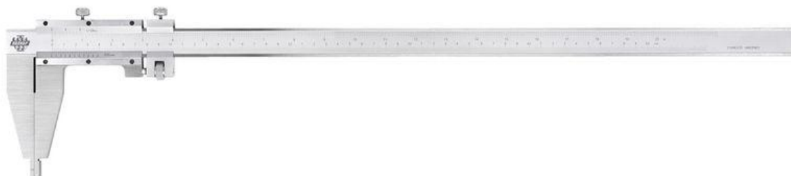
Рисунок 6 – Общий вид штангенциркулей типа ШЦ-III
