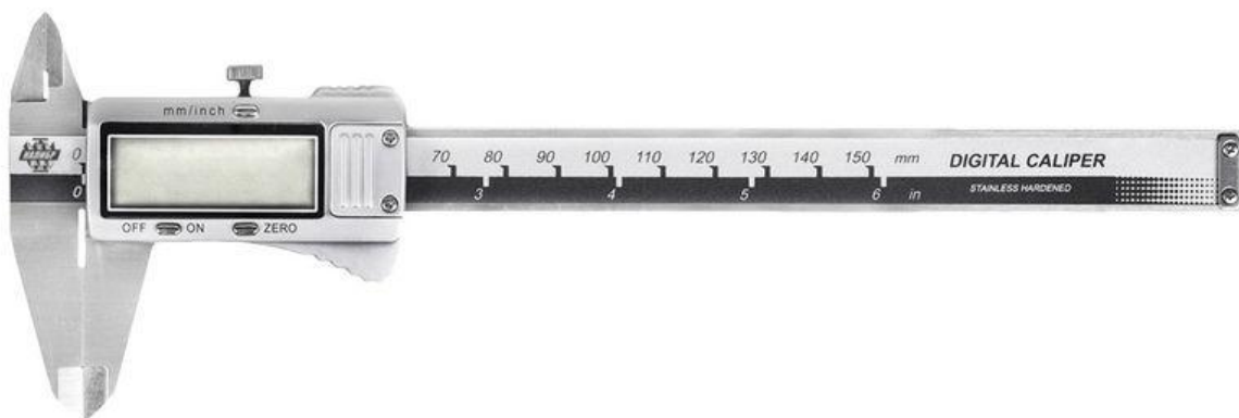
Рисунок 3 – Общий вид штангенциркулей типа ШЦЦ-I
