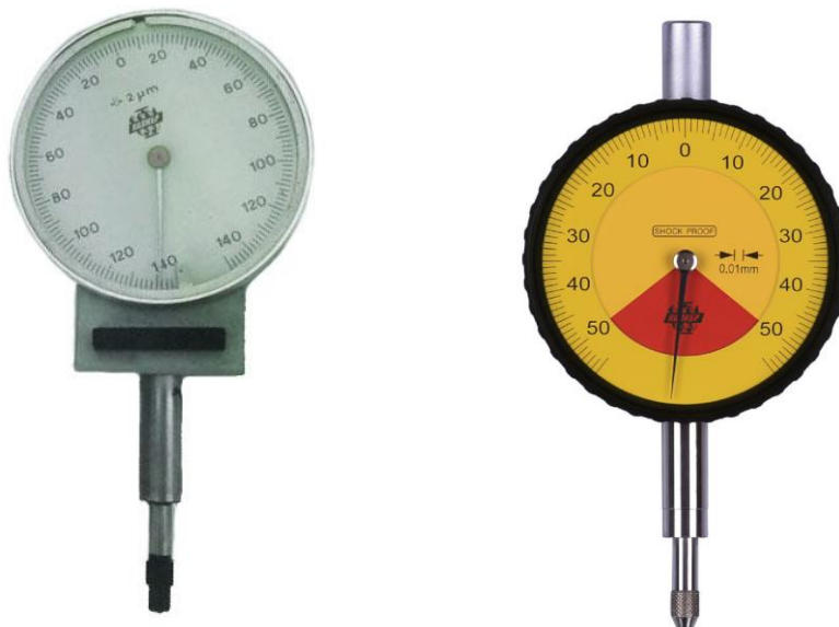
Рисунок 13 – Общий вид индикаторов часового типа моделей ИГ
